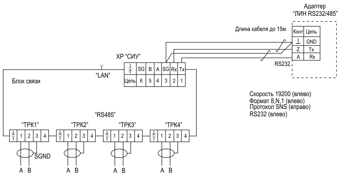
Схема подключения ТПК и уровнемера ПМП-201 по интерфейсу RS-232 к БС
