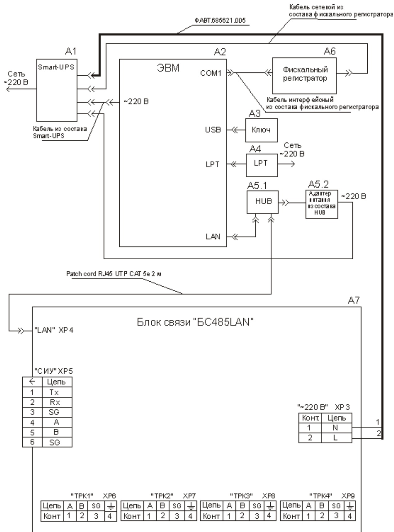
Схема соединений ПТК АЗС
